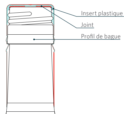
Stelvin® Lux / Stelvin® Lux+
